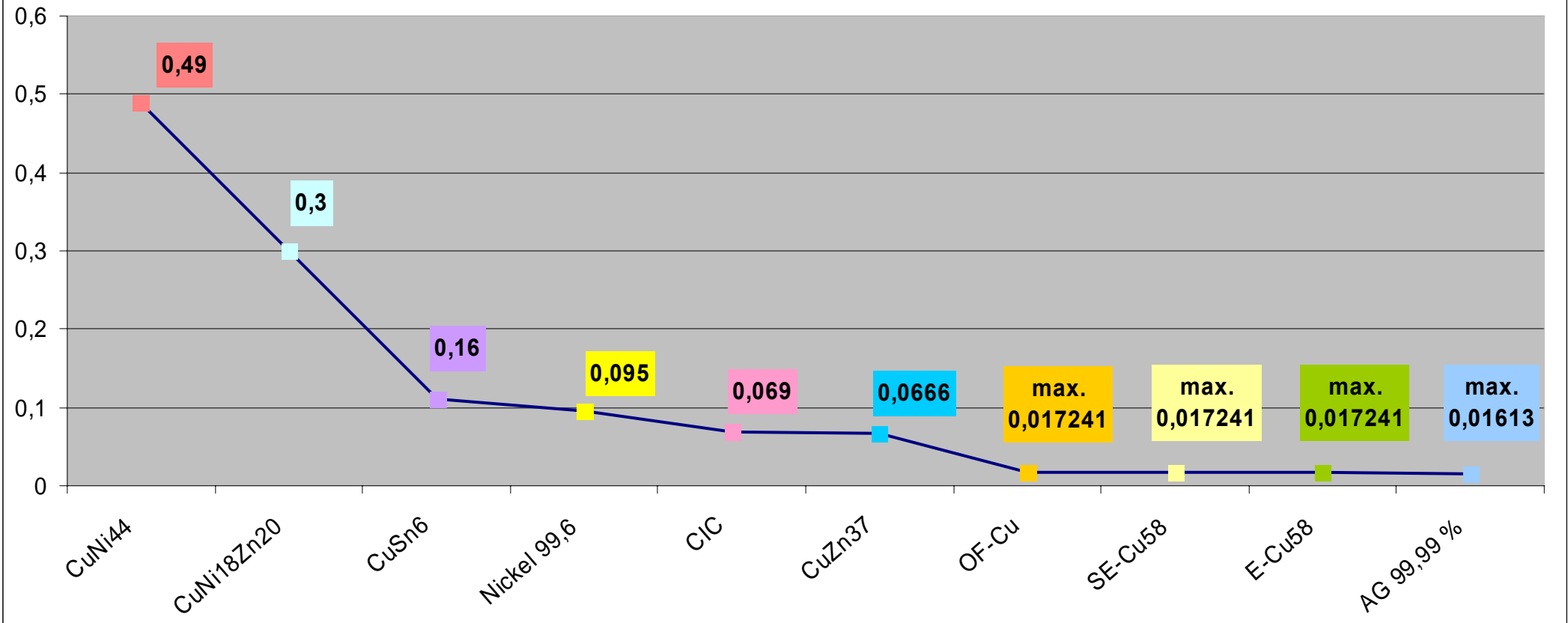
spezifischer elektrischer Widerstand \Omega \text{ mm}^2/\text{m}
